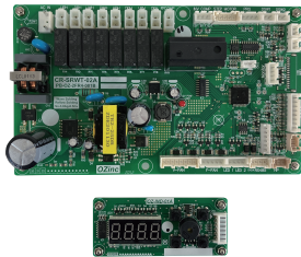
制御基板 Model No. : CR-SRWT-02A
